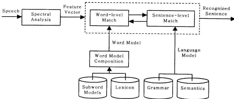
그림 2. 대어휘 연속음성 인식기 기본 구조
