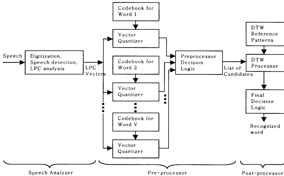
그림 1. 소어휘 고립단어 인식기 구현 예제
