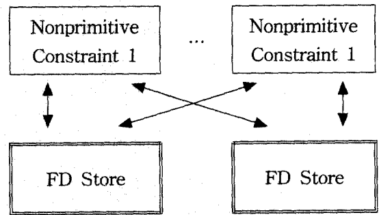
〈그림 3〉 하이브리드 솔버의 제약식 저장고와 비원시제약식
