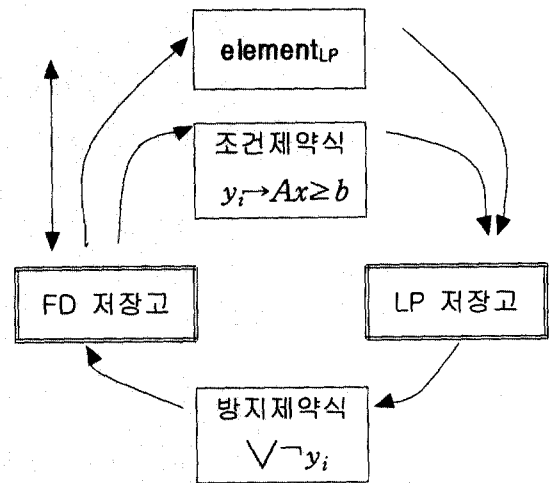
〈그림 4〉 하이브리드 솔버의 비원시 제약식들
