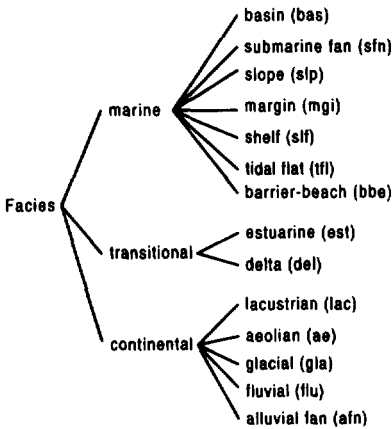
(그림 3) Facies 구조
